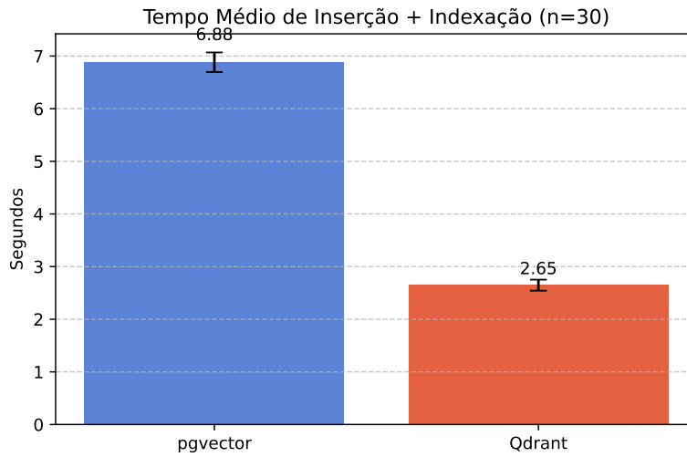
Figura 6. Comparativo do tempo médio de inserção e construção do índice HNSW ( n = 30 ). As barras de erro indicam o desvio padrão observado.
