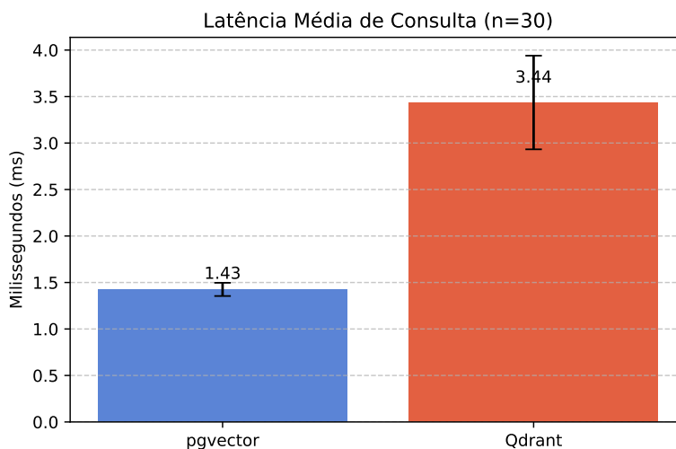
Figura 7. Comparativo da latência média por consulta ( k = 10 ). As barras de erro evidenciam a maior variância na comunicação com o Qdrant.
